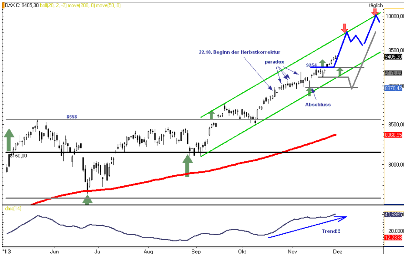
DAX Tageschart
